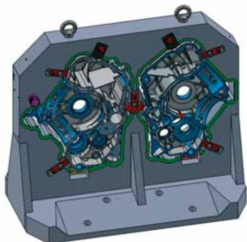
Mechanický upínací přípravek
