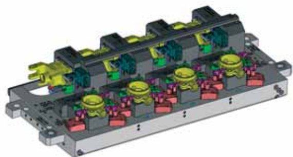
Hydraulický upínací přípravek
